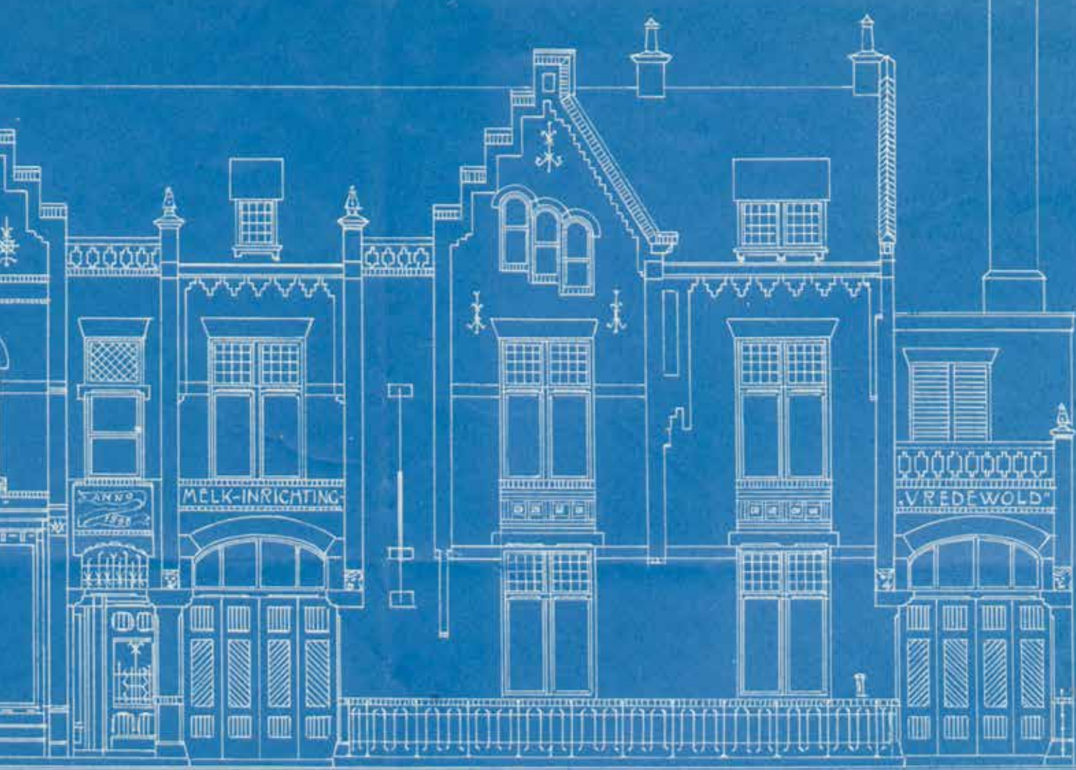
· DOORSNEDE · OVER · C-D ·
